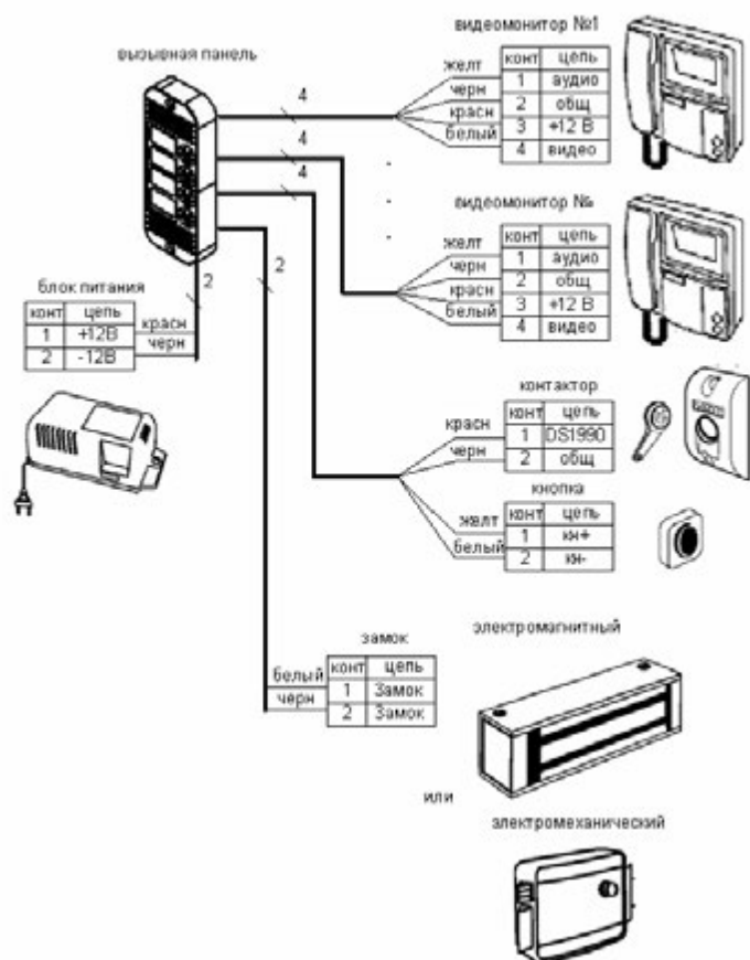
Рисунок 3.1 Схема подключения вызывной панели
