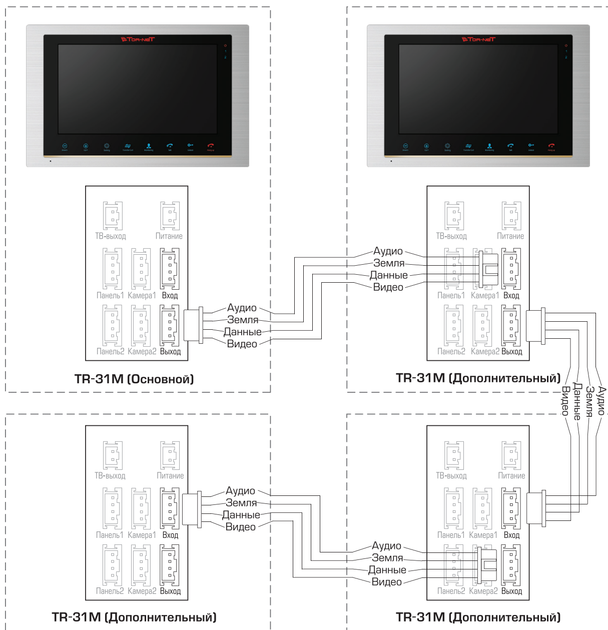
Схема 2. Подключение системы мониторов TR-31M
