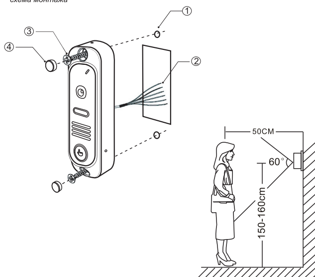
схема монтажа
