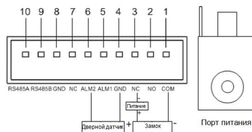
Электромагнитный замок
