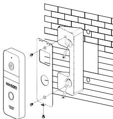
Рис. 5 Установки видеопанели под углом
