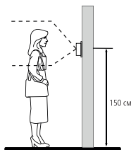
Рис. 3 Рекомендуемая высота установки видеопанели
