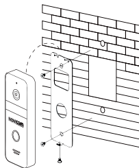
Рис. 4 Фронтальная установки видеопанели
