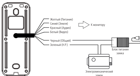
Рис. 2 Схема подключения видеопанели
