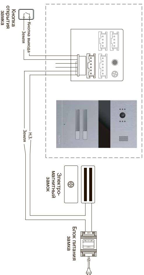
Схема 3. Подключение электромагнитного замка к панели МА-02.
