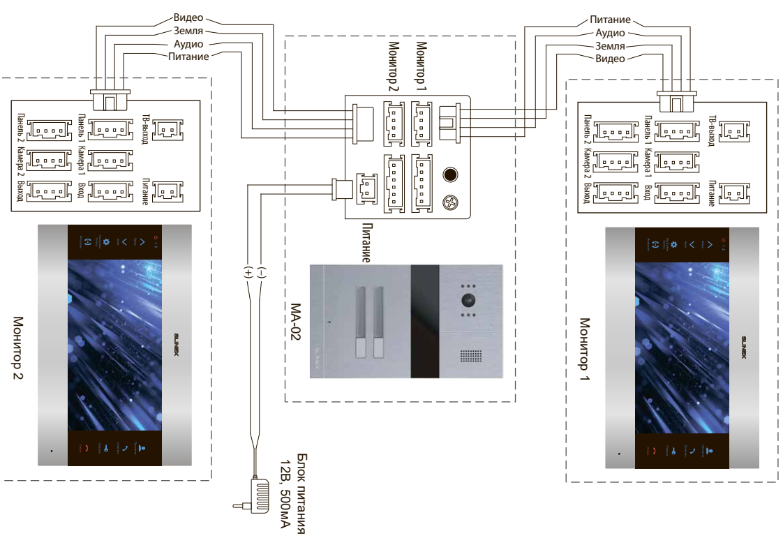
Схема 1. Подключение MA-02 с двумя мониторами.
