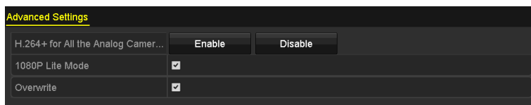
Рисунок 5-35 Расширенные настройки (для HQHI и HGHI-F серий DVR)
