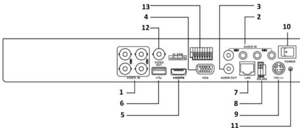
Рисунок 1-6 Задняя панель 2
