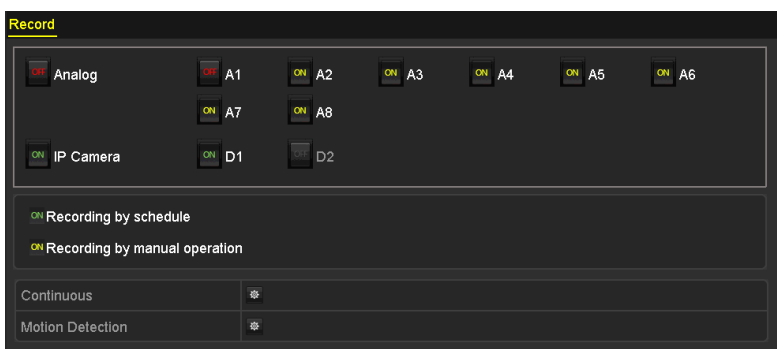
Рисунок 5-23 Запись вручную
