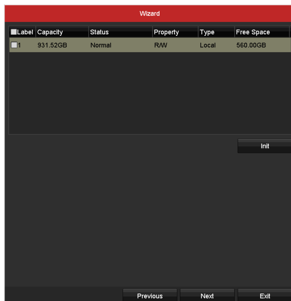
Рисунок 2-24 Управление HDD
