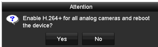
Рисунок 5-37 Предупреждающее окно
