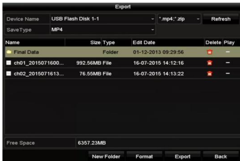
Рисунок 7-9 Управление устройствами хранения
