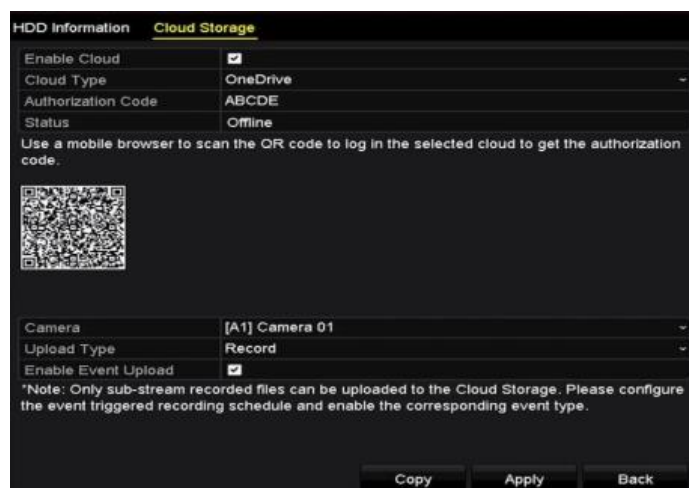
Рисунок 14-19 Меню настройки облачного хранилища
