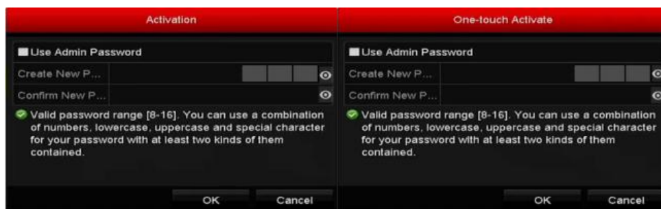
Рисунок 2-36 Активация камеры
