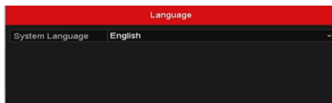
Рисунок 2-16 Настройка языка
