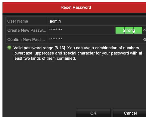
Рисунок 2-31 Сброс пароля
