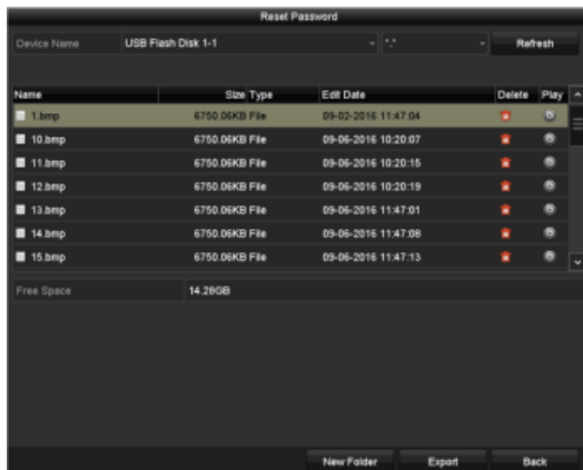
Рисунок 16-16 Экспорт GUID
