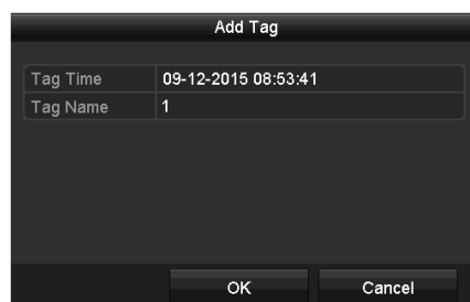
Рисунок 6-10 Добавление метки
