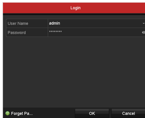
Рисунок 2-27 Меню входа
