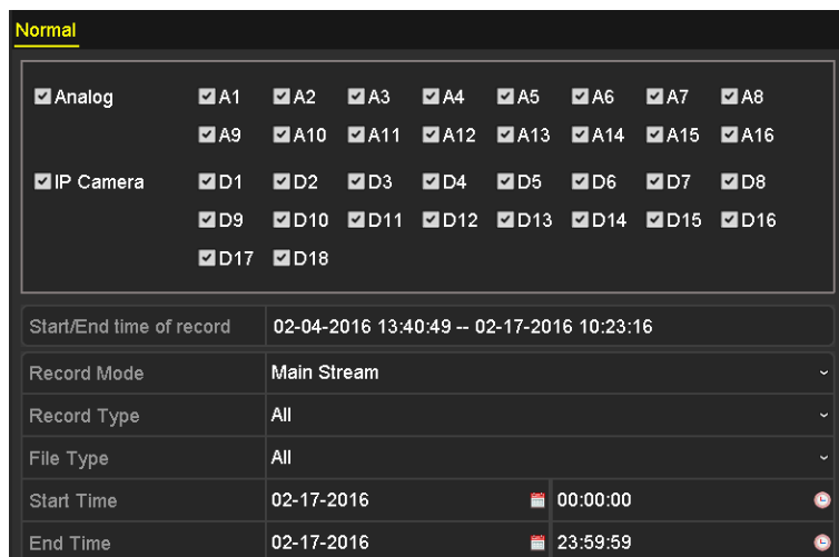
Рисунок 5-31 Экспорт
