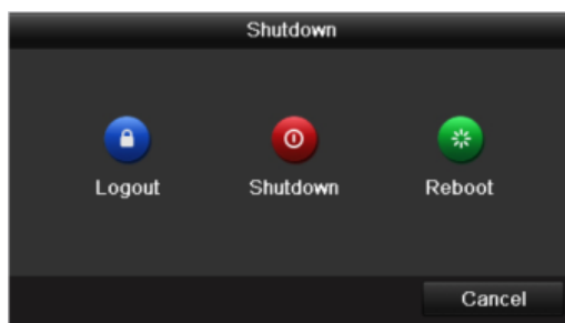
Рисунок 2-1 Меню выключения
