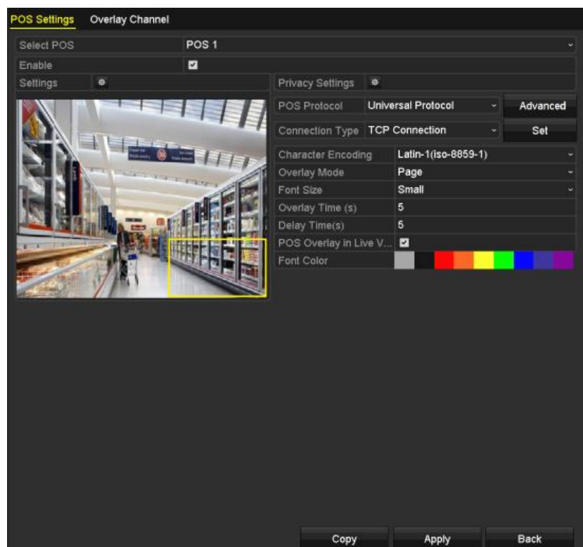
Рисунок 9-1 Настройки POS
