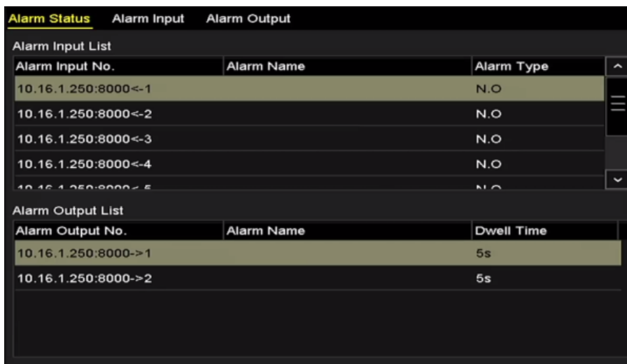
Рисунок 5-17 Настройки тревог
