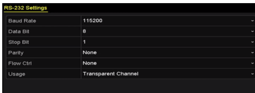
Рисунок 9-10 Настройки RS-232
