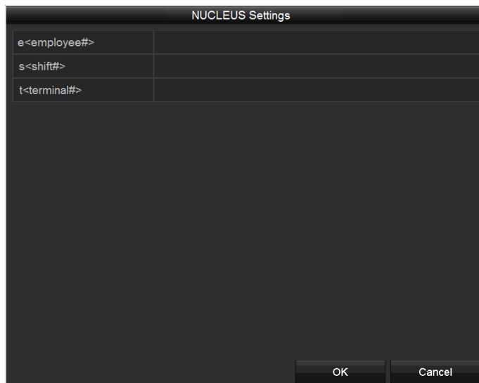
Рисунок 9-5 Настройки NUCLEUS
