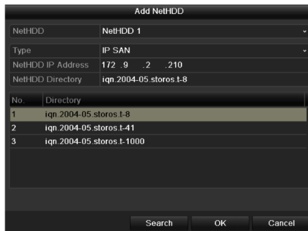
Рисунок 14-9 Добавление IP SAN диска
