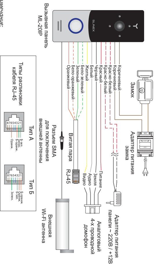
Схема 1. Подключение питания и замка к панели МЛ-201Р.
