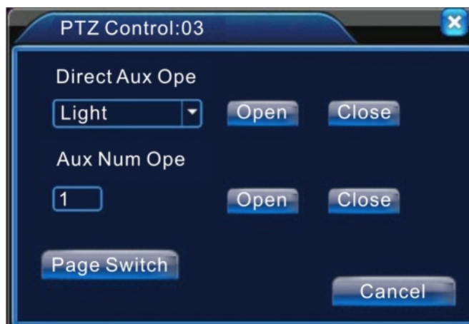
Рис 3.17. Вспомогательные настройки
