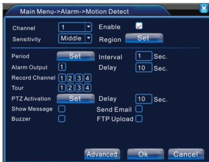
Рис 4.4. Детекция движения
