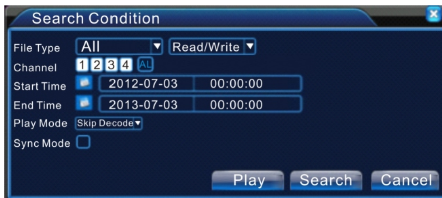
Рис 3.7. Отбор записей
