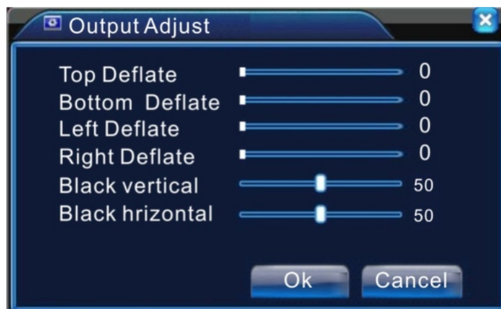
Рис 3.19. Калибровка экрана
