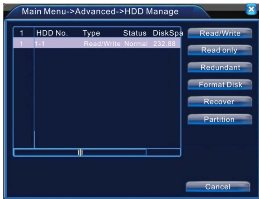
Рис. 4.33. Управление НЖМД
