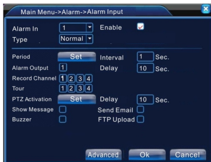
4.10. Вход тревоги
