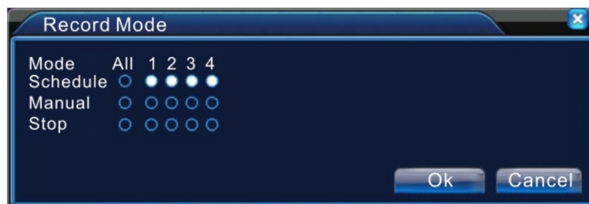
Рис 3.8. Режимы записи
