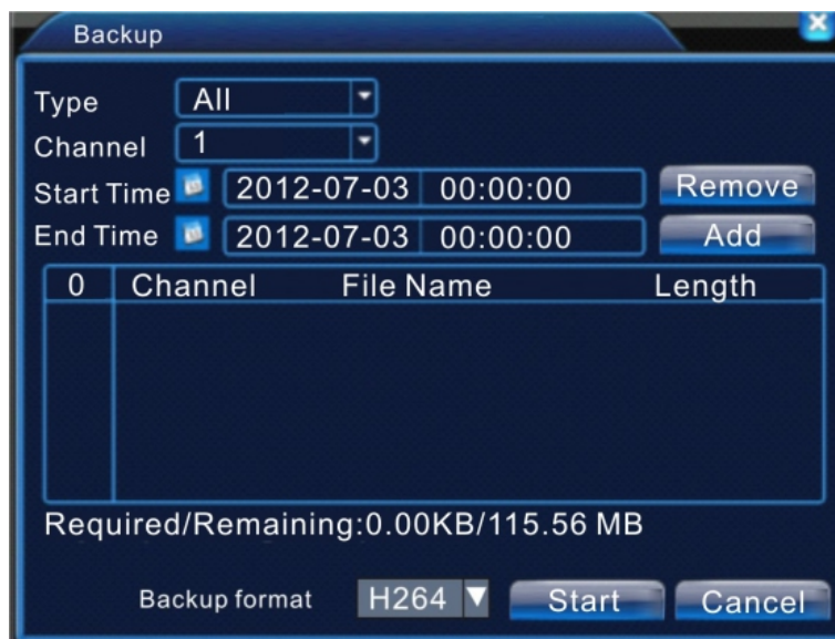
Рис 4.3. Архивация файлов
