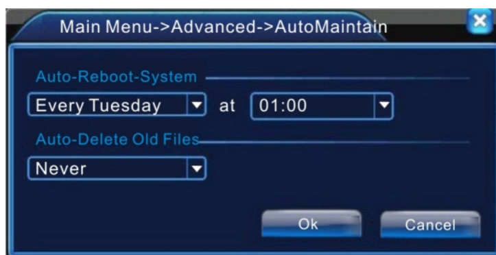
Рис. 4.41. Автоматические функции
