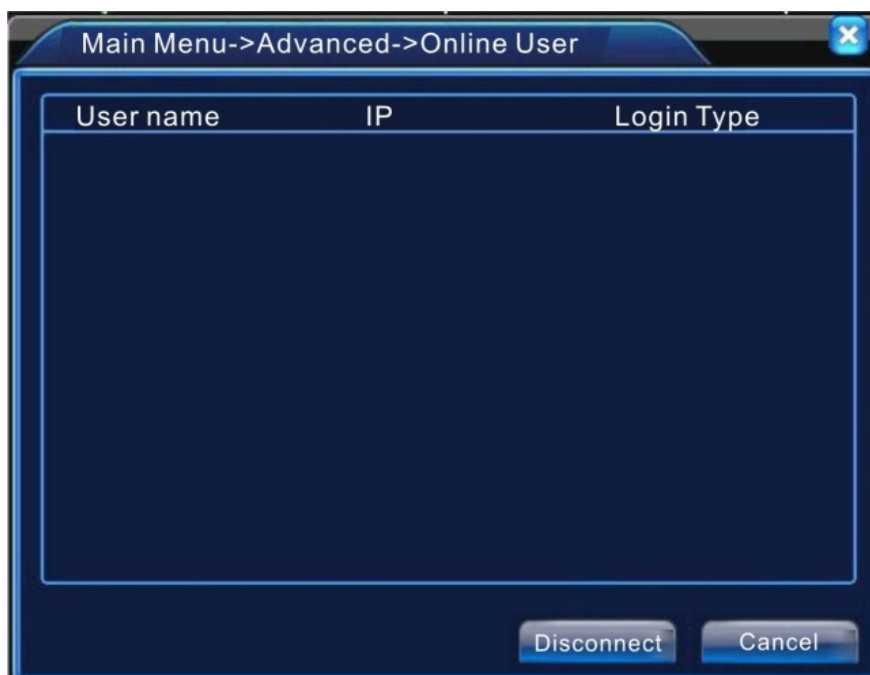
Рис. 4.40. Пользователи
