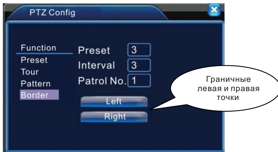
Рис 3.16. Настройки автосканирования
