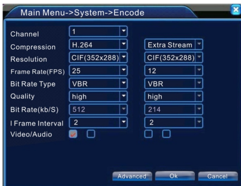
Рис 4.15. Настройки кодирования
