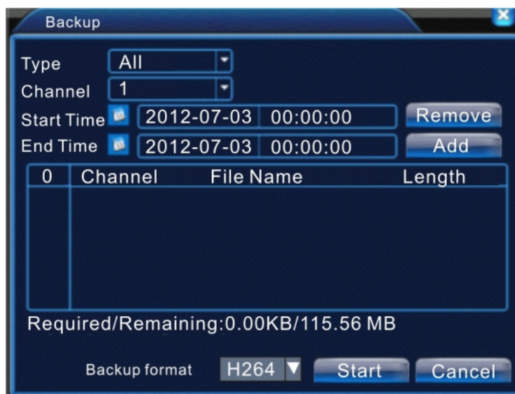
Рис 3.6. Архивация
