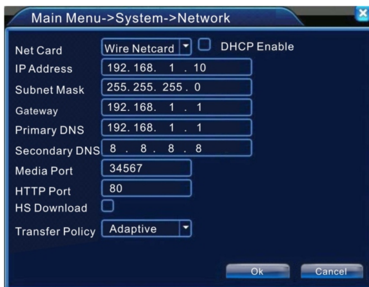
Рис 4.16. Настройки сети
