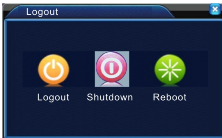
Рис 3.20. Выход
