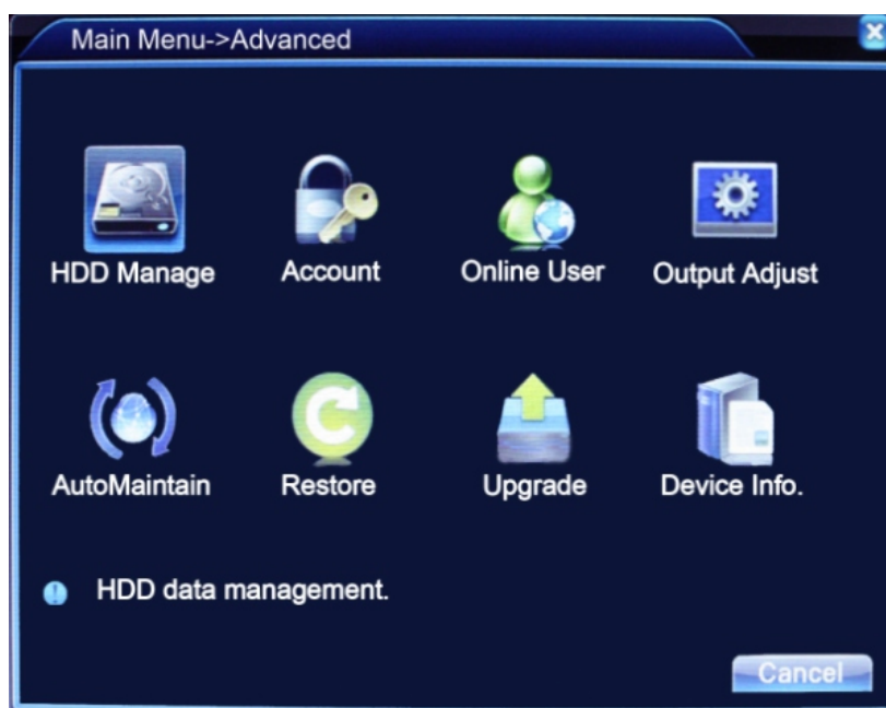
Рис. 4.32. Управление
