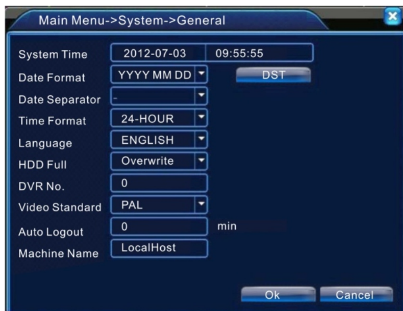
Рис 4.12. Общие настройки
