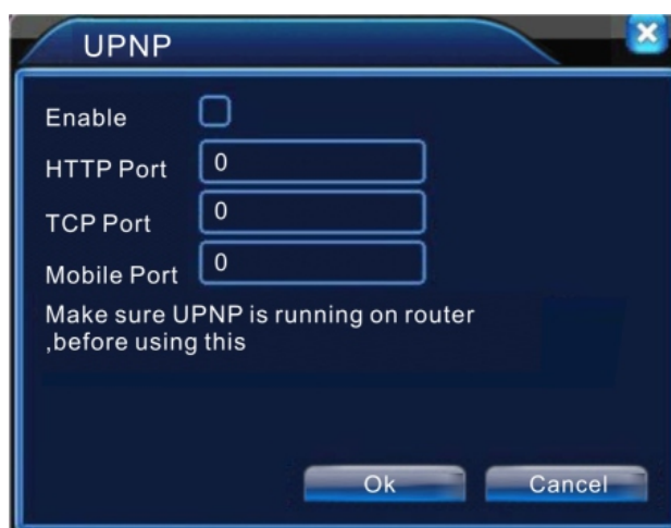
Рис 4.27. Настройка UPnP
