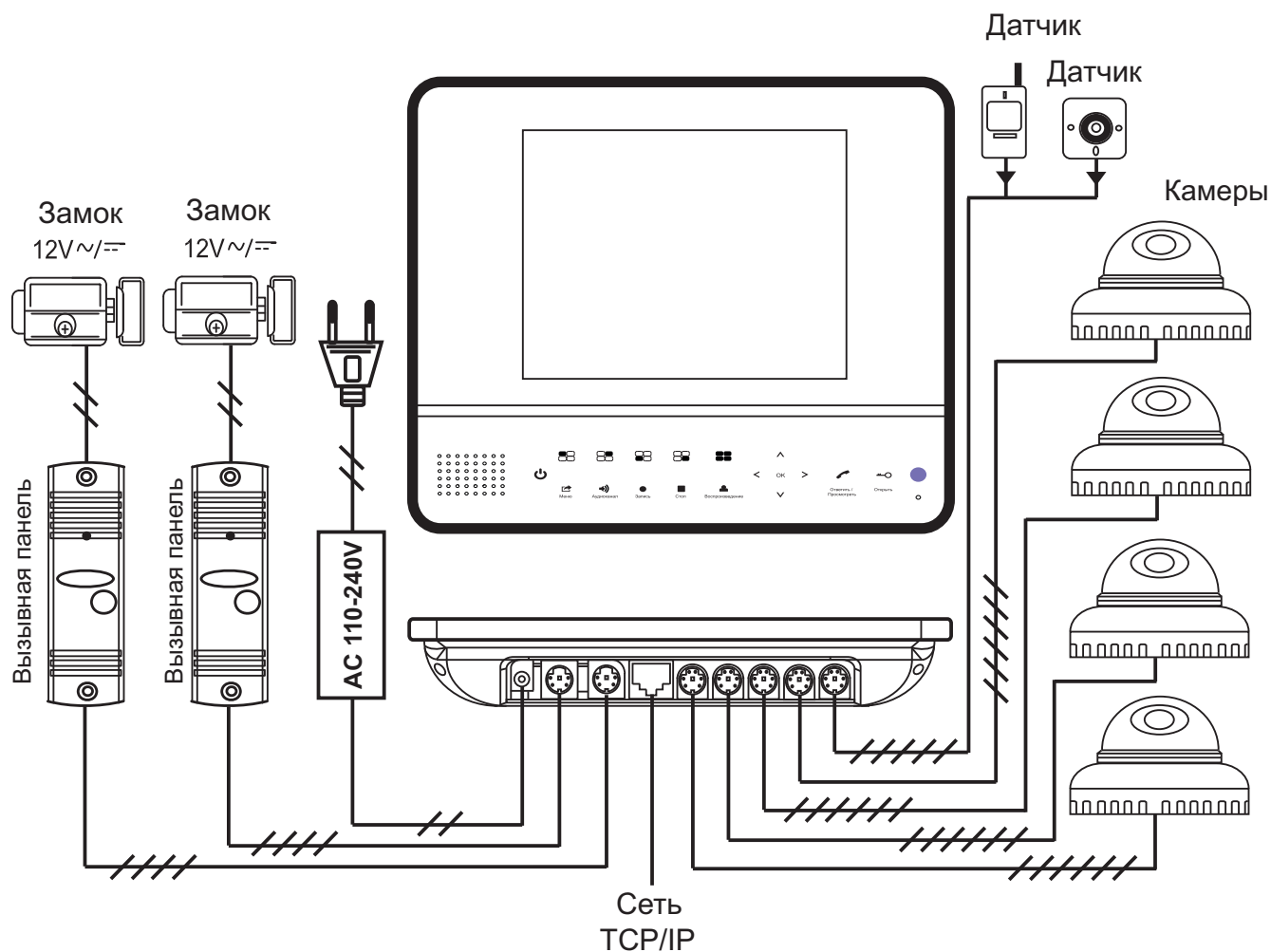
Рис 2.5. Подключение монитора
