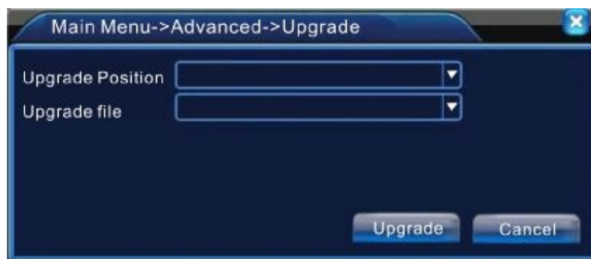
Рис. 4.43. Обновление
