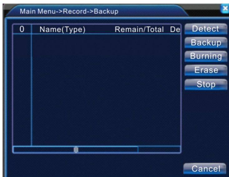
Рис 3.5. Поиск накопителя
