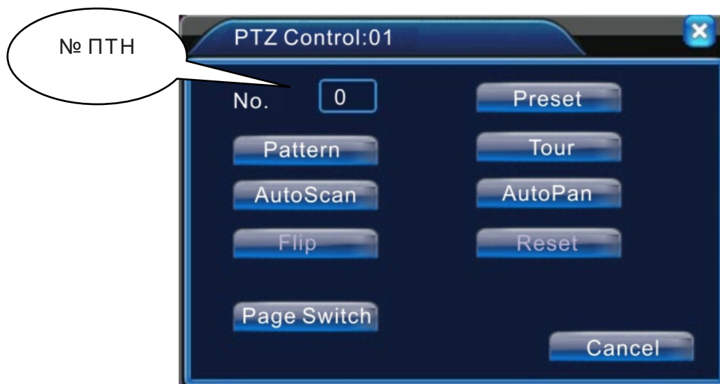
Рис 3.13. Управление PTZ
