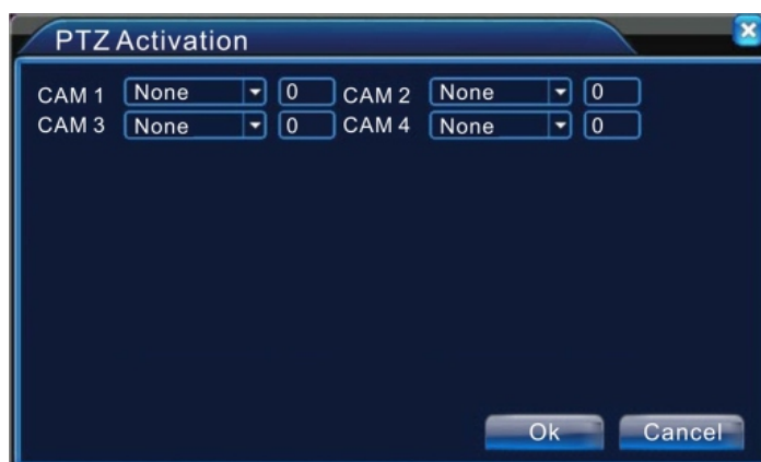
Рис 4.7. Включение PTZ
