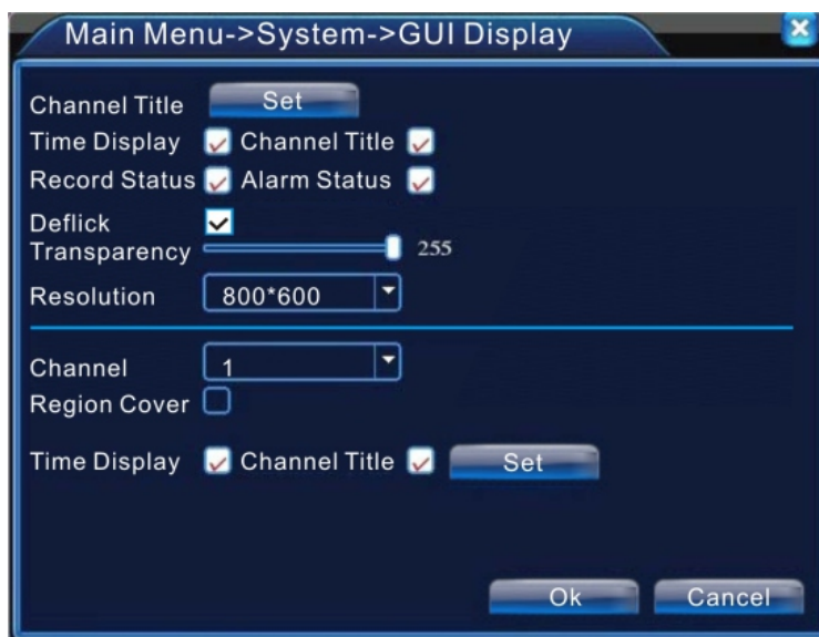
Рис 4.28. Дисплей
