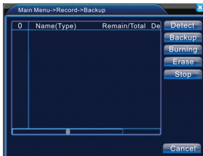
Рис 4.2. Поиск накопителей
