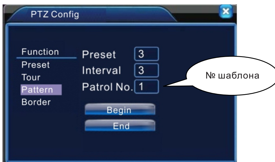
Рис 3.15. Настройка шаблонов
