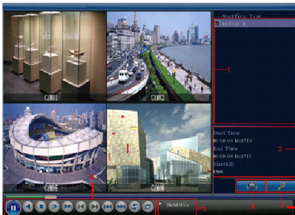
Рис 3.4. Воспроизведение
