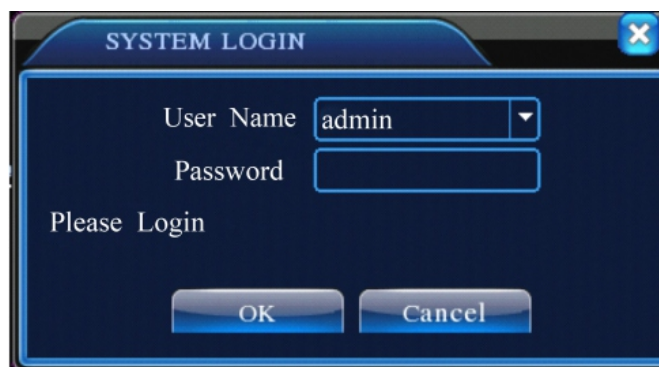
Рис 3.1. Авторизация
