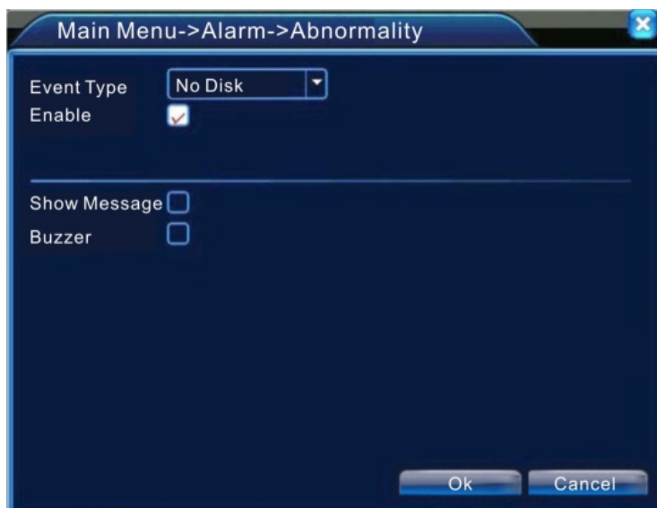
Рис 4.11. Лог ошибок
