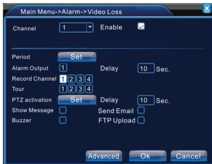
4.9. Потеря видеосигнала
