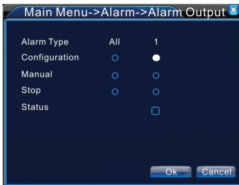
Рис 3.10. Выходы тревоги
