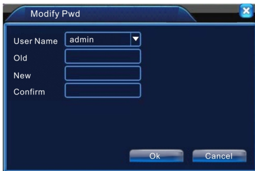
Рис. 4.35. Изменение пароля
