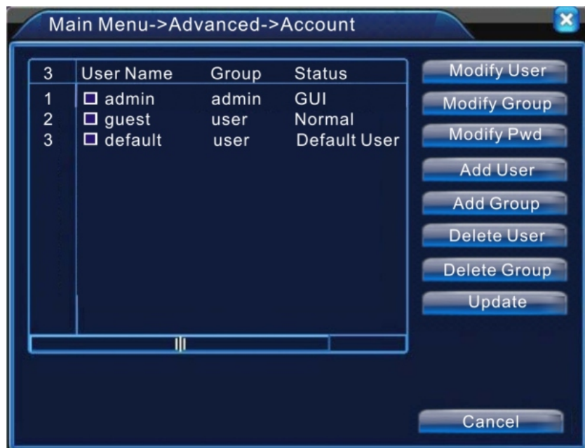
Рис. 4.34. Учетные записи
