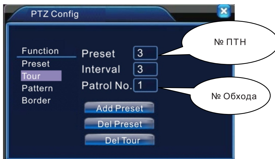
Рис 3.14. Настройки обходов
