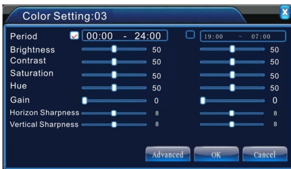
Рис 3.18. Настройка цвета
