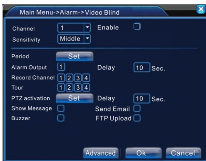
Рис 4.8. Закрывание изображения
