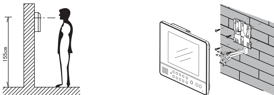
Рис. 2.5. Установка монитора
