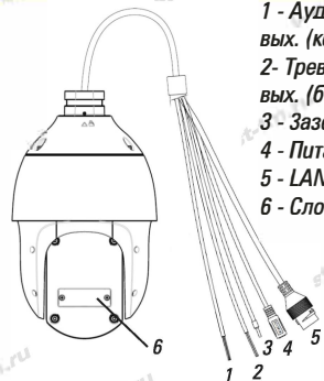
Рис.1 Схема подключения
