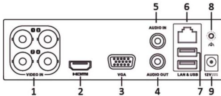
Рисунок 1-5 Задняя панель 1
